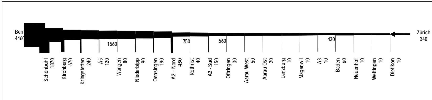
Verkehrs-Struktur A1: In BERN von Richtung ZÜRICH aus ankommender Verkehr (Fz/h)
